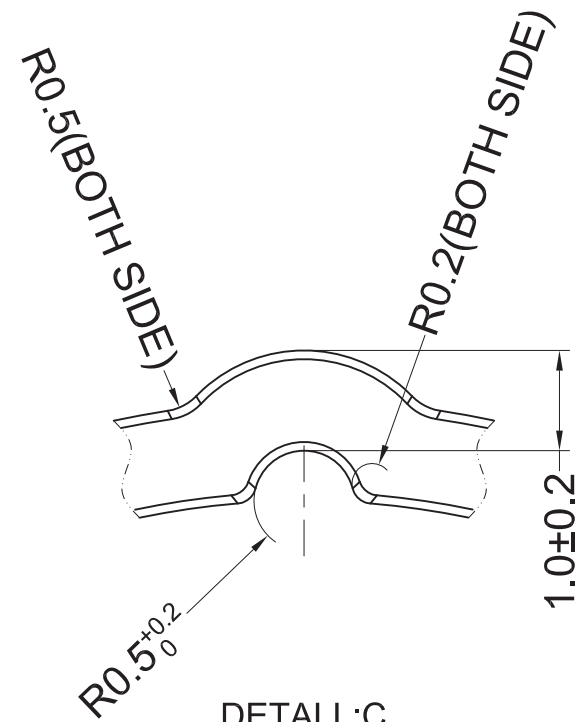
DETAIL:C (5:1)
